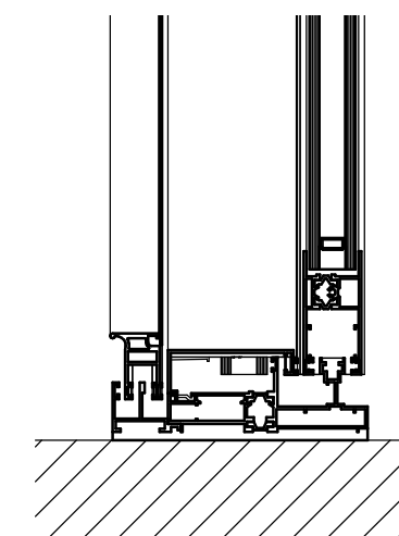
7 Detail 5 1 : 5
