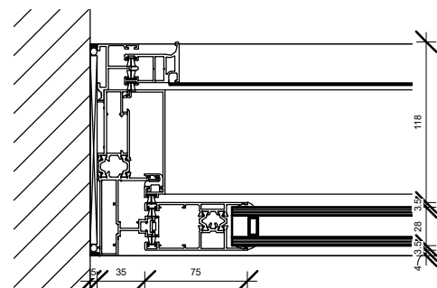
3 Detail 1 1 : 5
