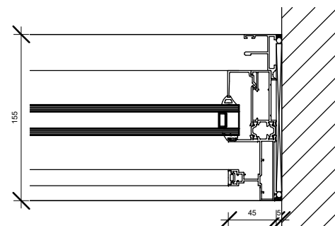
5 Detail 3 1 : 5
