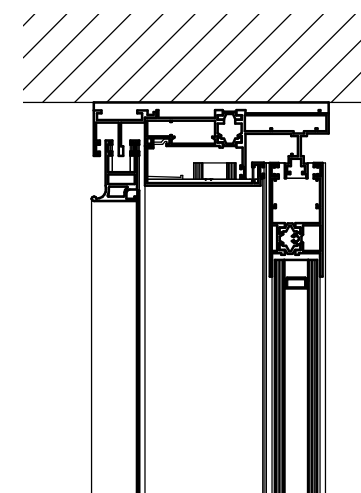
6 Detail 4 1 : 5
