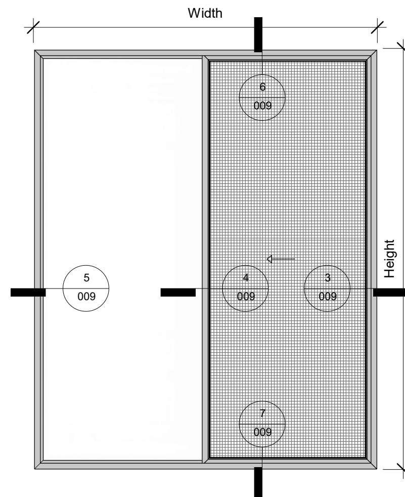
2 Elevation Back 1 : 20
