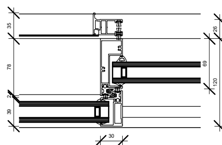
4 Detail 2 1 : 5
